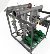
Насосные станции
